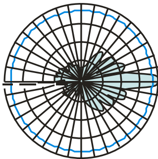
E-plane
