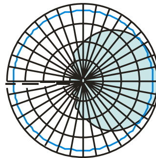
H-plane
